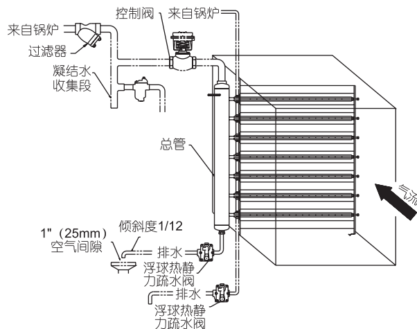
图139-3 HumidiPackPlus® “增强格栅式加湿器”
